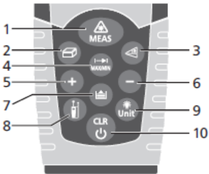
Abb. 1: Gerätebeschreibung
