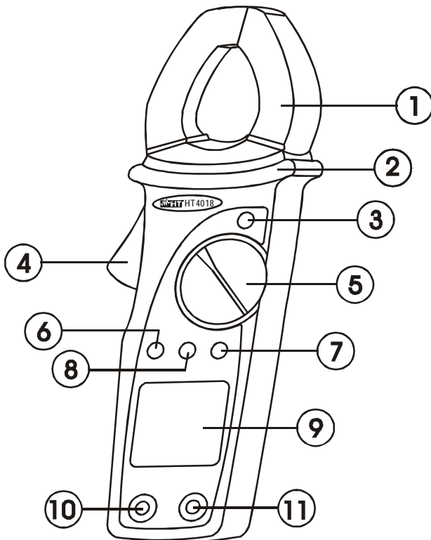
Abb. 1: Instrumentenbeschreibung
