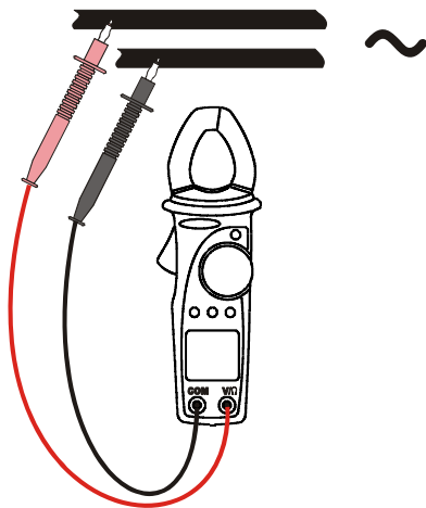
Abb. 4: AC Spannungsmessung
