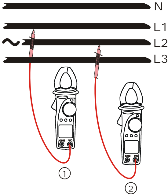
Abb. 14: Messung der Phasenfolge
