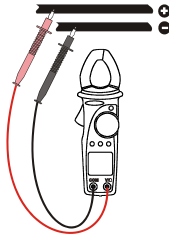
Abb. 5: DC Spannungsmessung
